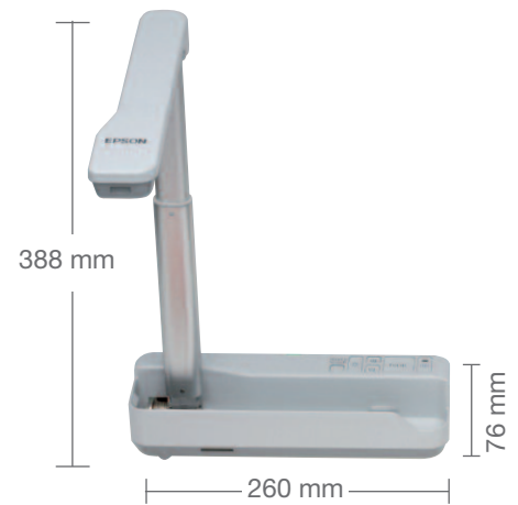
Abmessungen (aufgeklappt)
