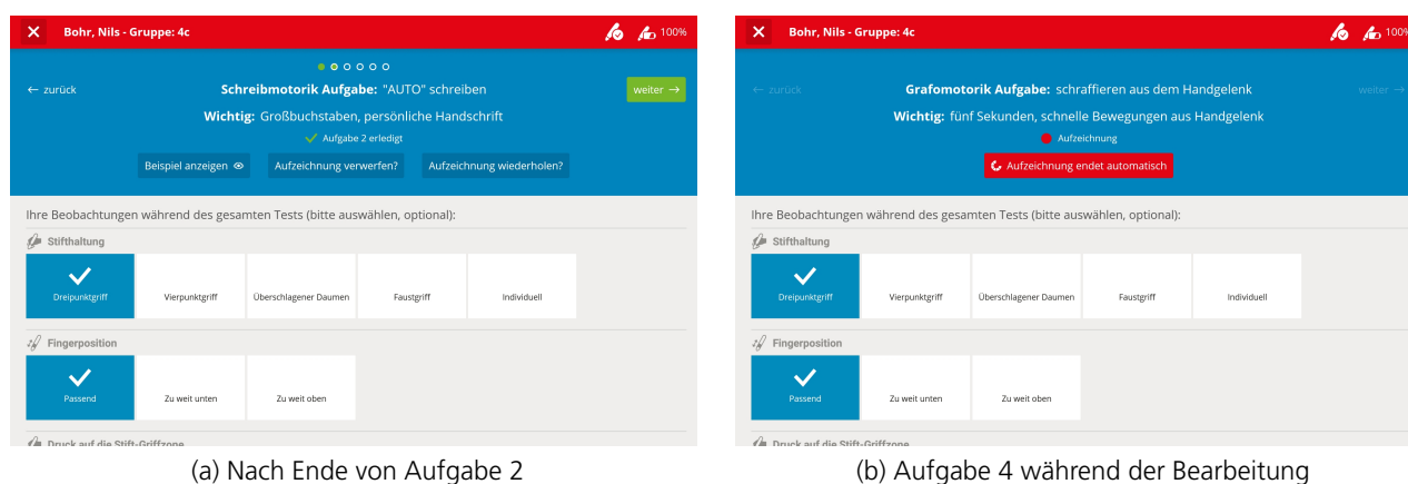
Abbildung 20: Testaufgaben
