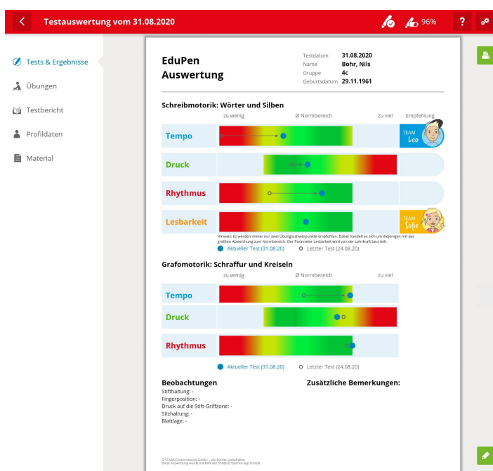
Abbildung 22: Testauswertung
